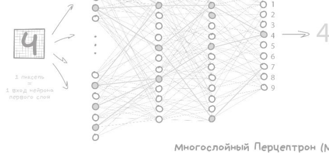
Многослойный Перцептрон (MLP)
